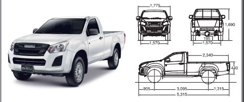
سيارة دفع رباعي بمقصورة مفردة - آر بي آيه
